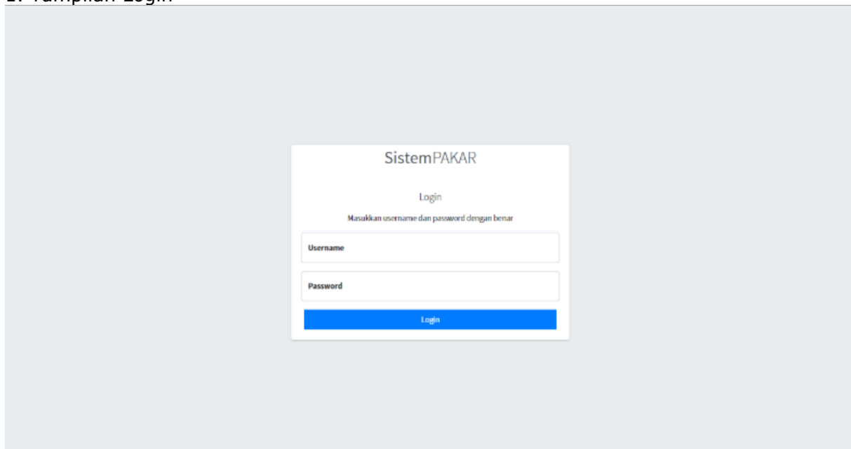
Gambar 5. Tampilan Login
